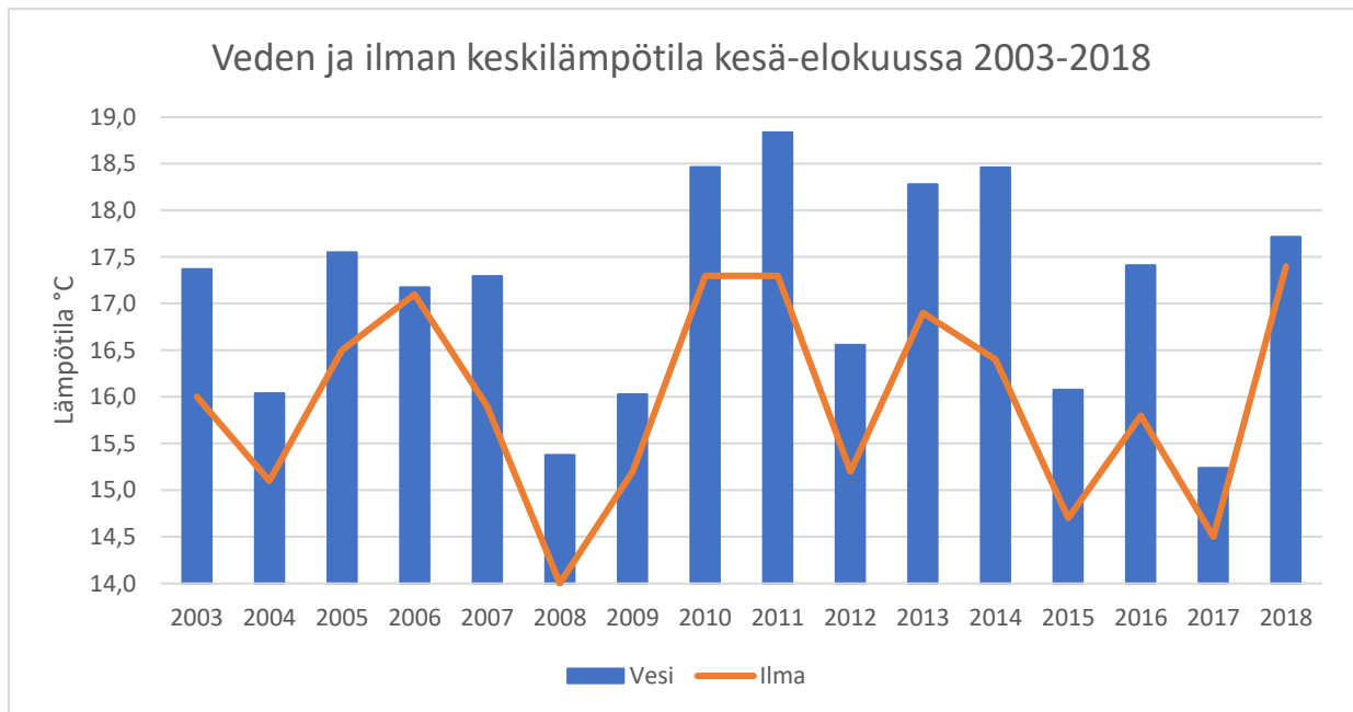
Kuva 2. Veden ja ilman lämpötilat kesä-elokuussa 2003-2018. Ilmanlämpötilat ilmatieteenlaitoksen Kuopion mittauspiste. Vedenlämpötilat Ympäristötiedon hallintajärjestelmä Hertta.
